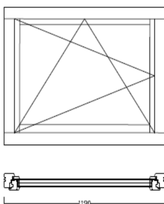
Kuva 1 DK-ikkunan periaatekuva (A-malli)
