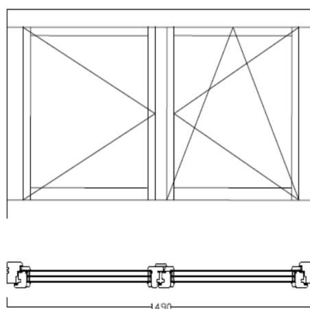
Kuva 2 DK-ikkuna kohtaavilla puitteilla (DK/2, B-malli)
